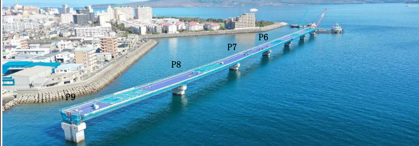
床版コンクリート打設完了(3回目)
