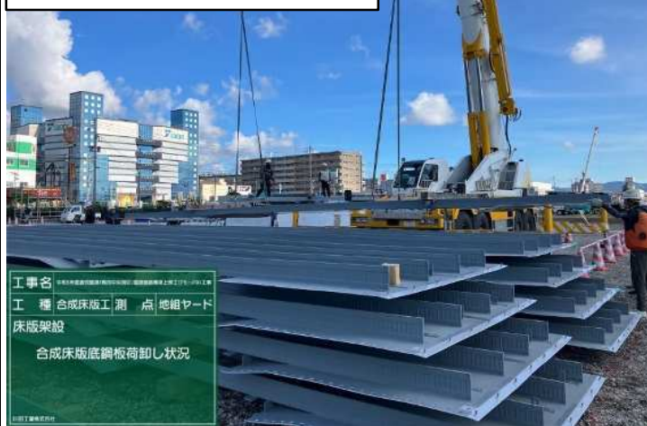
合成床版底鋼板荷卸し状況
