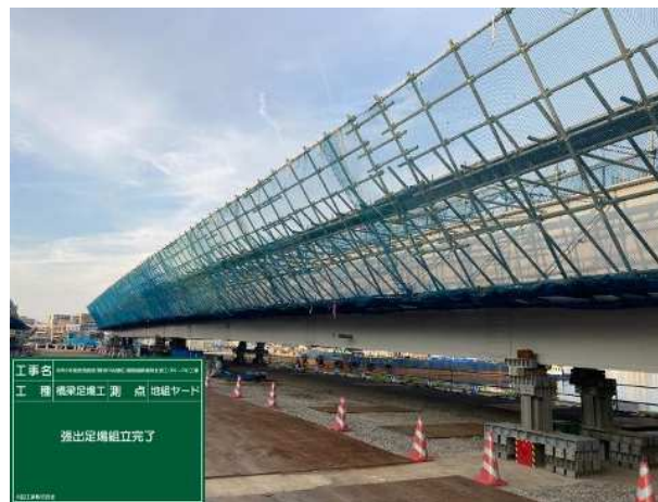
張出足場組立完了(5/15撮影)
