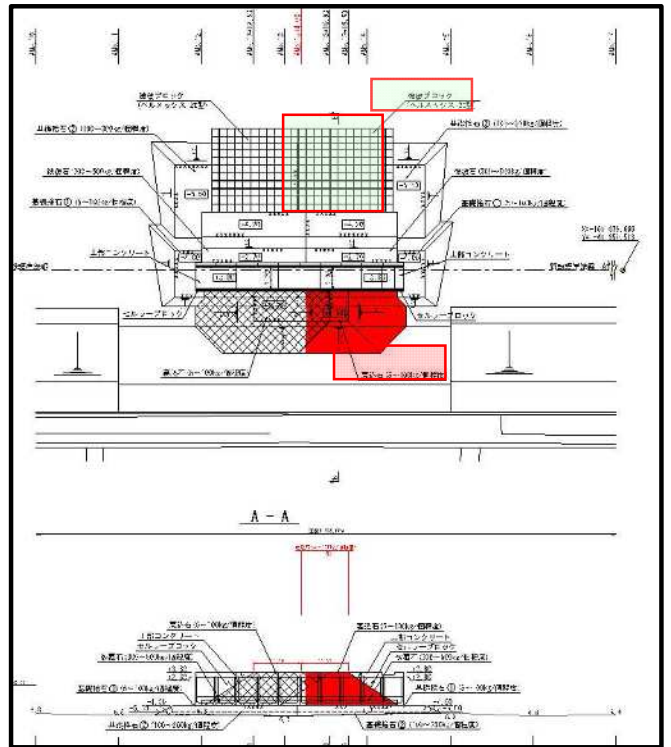
裏込材投入図 (雑石5~100kg/個程度) 被覆ブロック据付図 (2t型)
