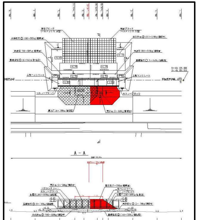
裏込材投入図 (雑石5~100kg/個程度)
