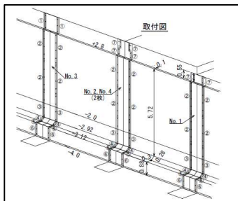
防砂目地板取付箇所 防砂目地板取付図
