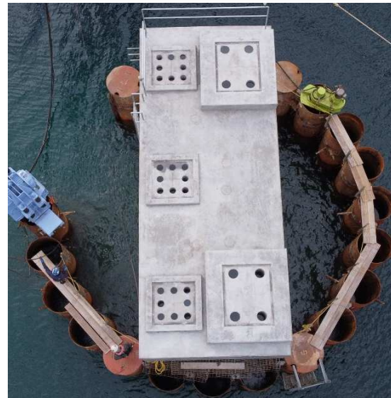
鋼管矢板切断・撤去状況
