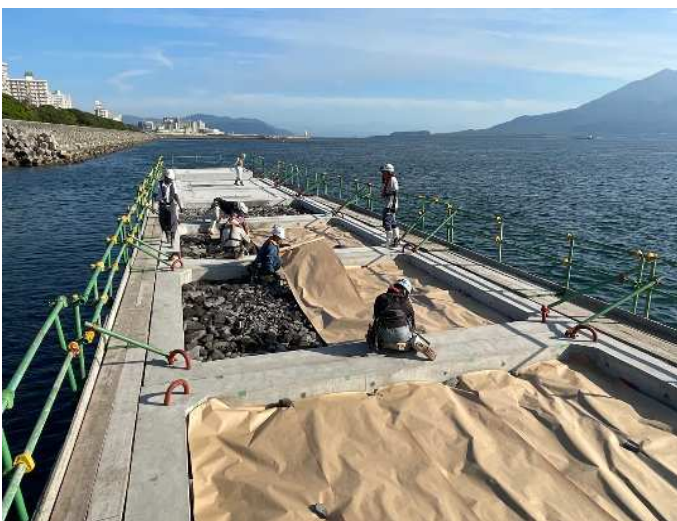
上部工①コンクリート打設準備
