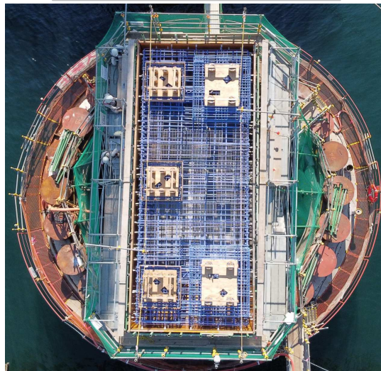
梁鉄筋・型枠組立完了
