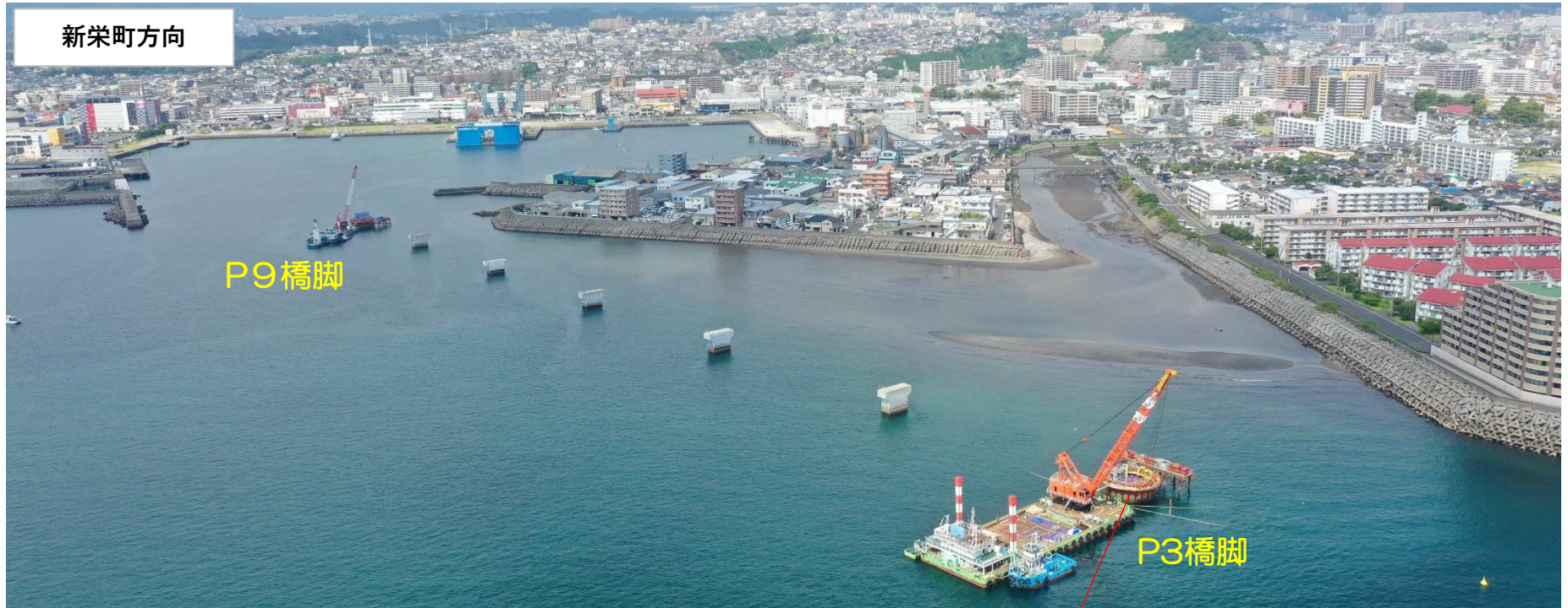
柱鉄筋組立状況 (令和5年9月27日撮影)
