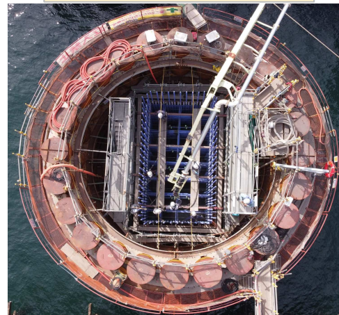
柱コンクリート打設状況 (令和5年10月13日撮影)
