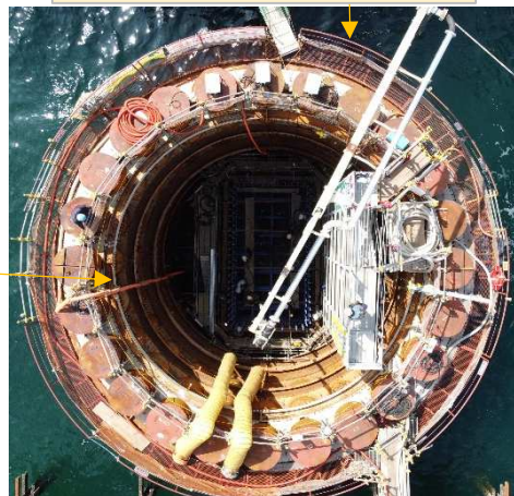
柱コンクリート打設状況 (令和5年9月13日撮影)
