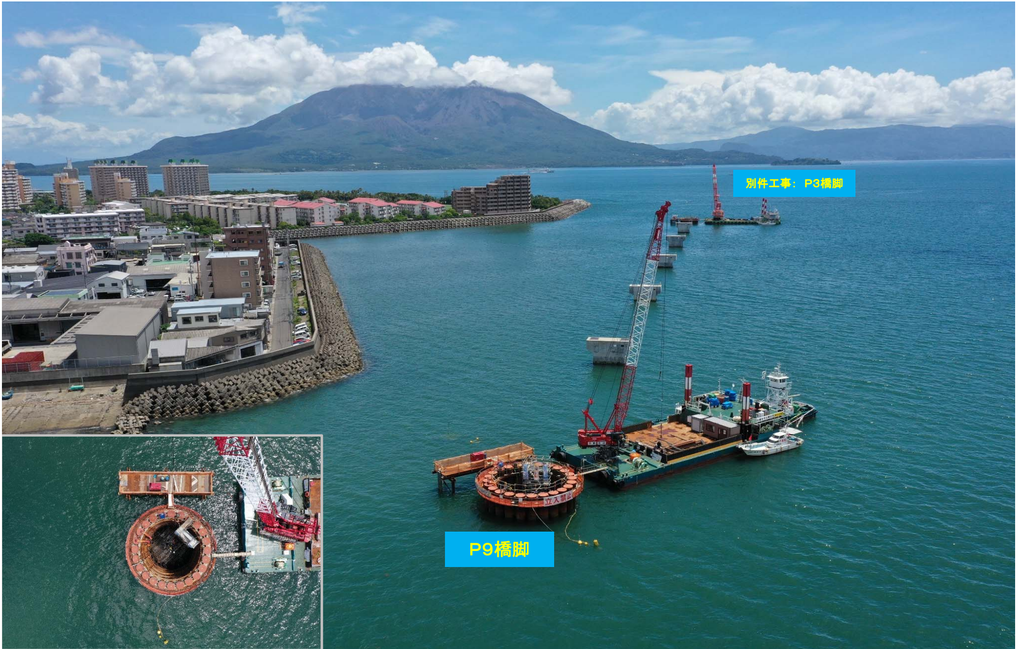
(令和5年6/27 撮影：頂版鉄筋組立状況 りんかい日産建設(株))
