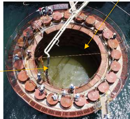
コンクリート打設状況
